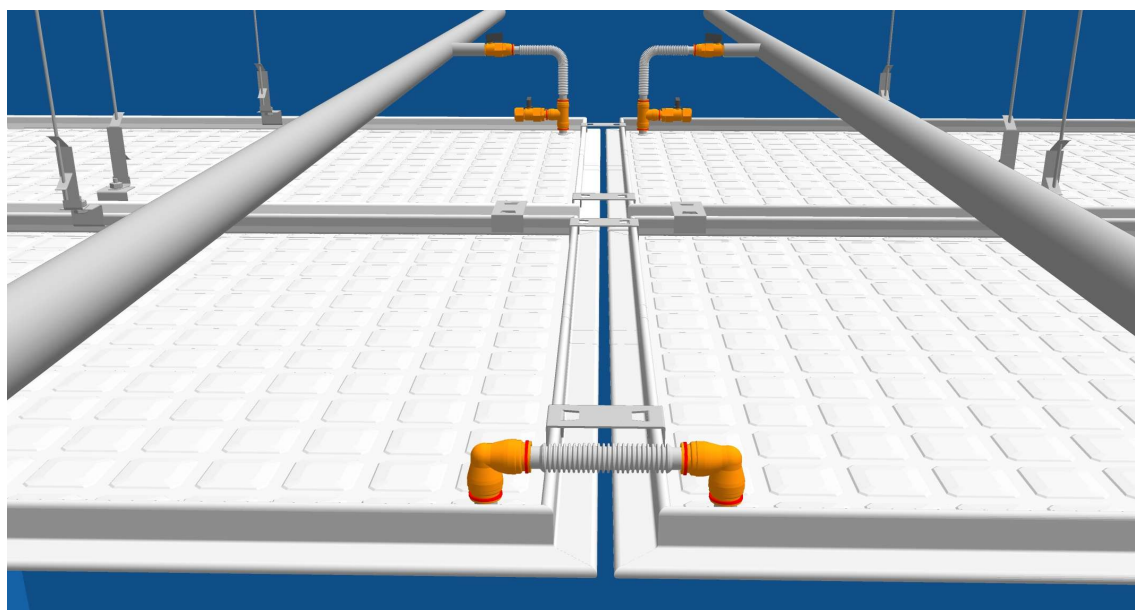
Fig. 6 – Raccordement hydraulique d'un îlot de panneaux climatiques (Kigo standard) avec les raccords rapides et les flexibles métalliques
