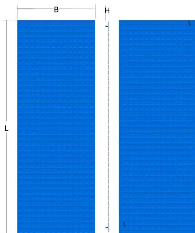
Fig. 2 – L'échangeur Kigo et ses dimensions principales
