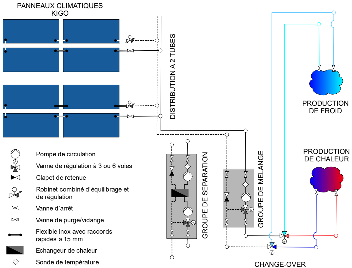
Fig. 8 – Distribution à deux tubes – schéma de principe
