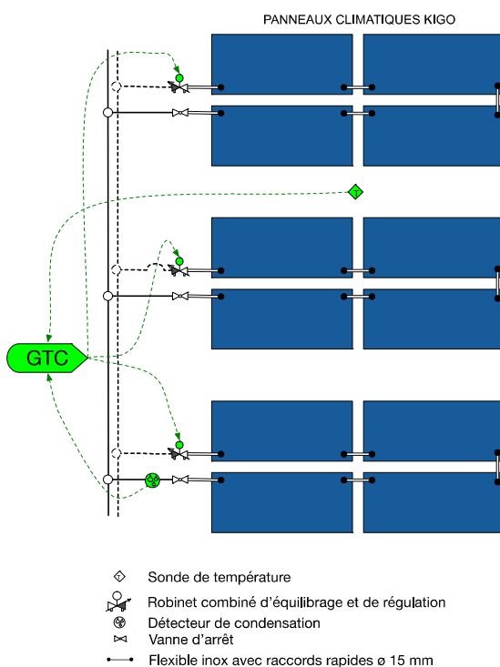
Fig. 13 – Réglage « modulaire » par îlot
