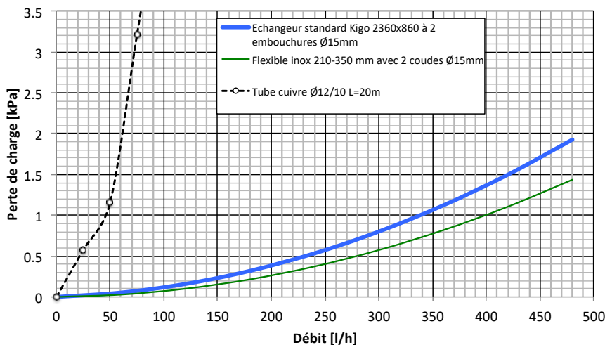
Fig. 4 – Perte de charge de l'échangeur Kigo
