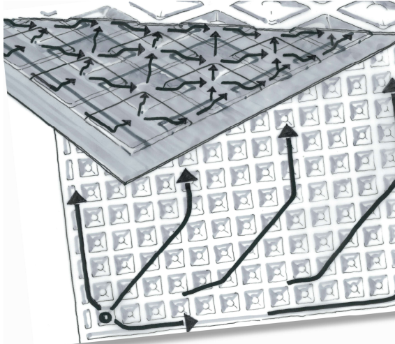
Fig. 1 - Concept de l'échangeur
