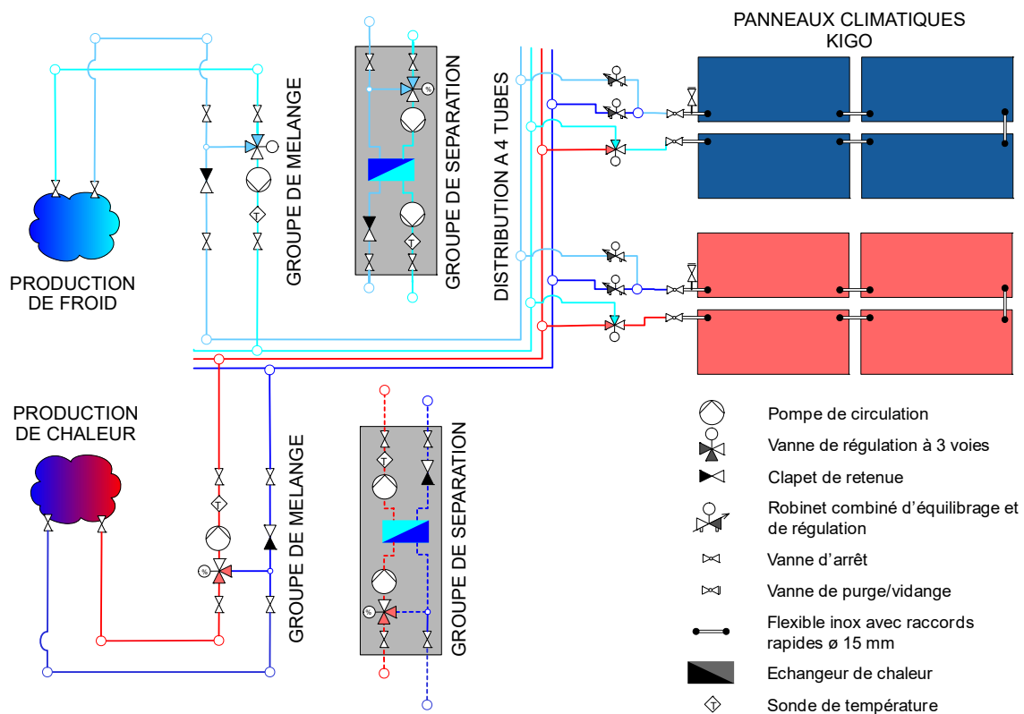
Fig. 9 – Distribution à quatre tubes – schéma de principe
