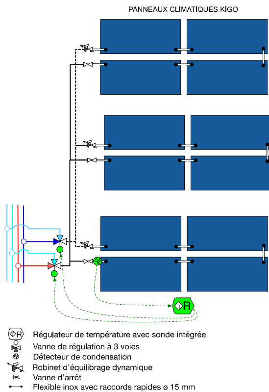
Fig. 12 – Réglage d'une zone comprenant plusieurs groupes
