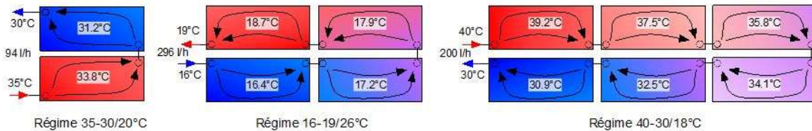
Fig. 5 – La création de groupes en « U » simplifie le raccordement hydraulique et assure une répartition homogène des températures
