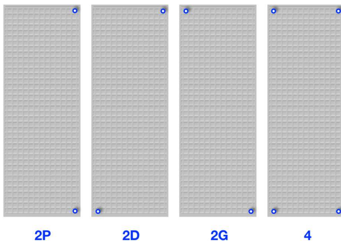
Fig. 3 – Dispositions possibles des embouchures
