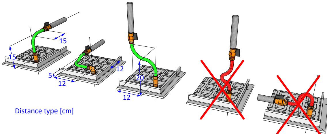
Fig. 7 – Flexibles de raccordement : en vert les géométries de raccordement adaptées et en rouge celles à exclure.
