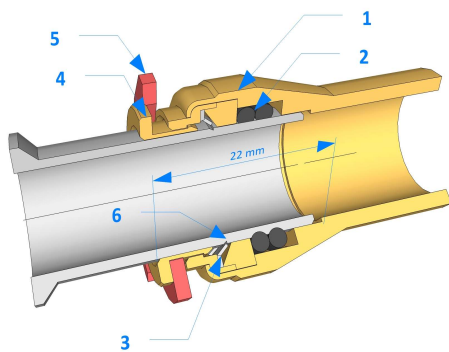
Fig. 5 - Design du raccord rapide
