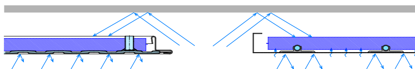
Fig. 7 - Akustisches Verhalten : LINKS Kigo Decke – RECHTS konventionelle Klimadecke
