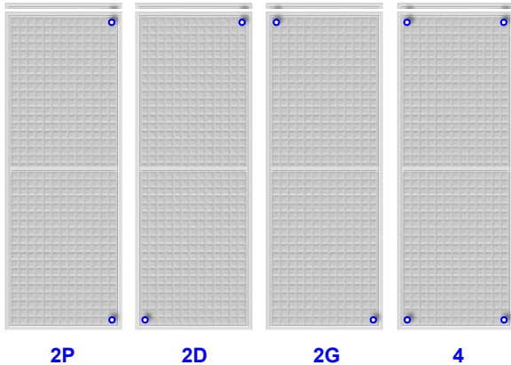
Fig. 4– Mögliche Anordnungen der Anschlüsse (Anblick auf der nicht sichtbaren Seite)
