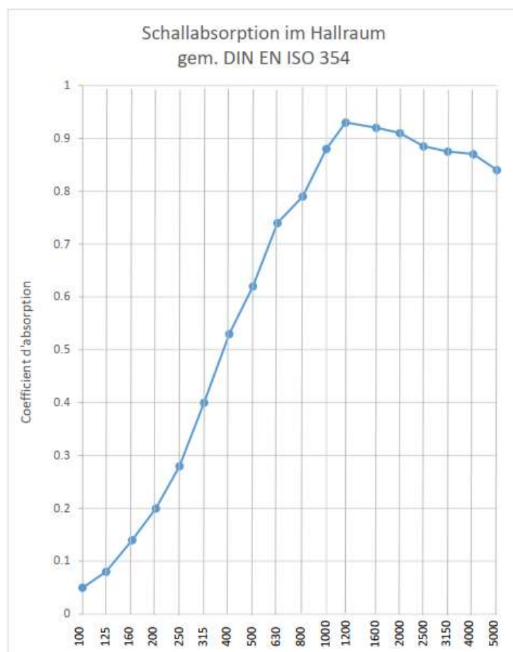
Fig. 9 - Absorptionskoeffizientenkurve Top-Phon
