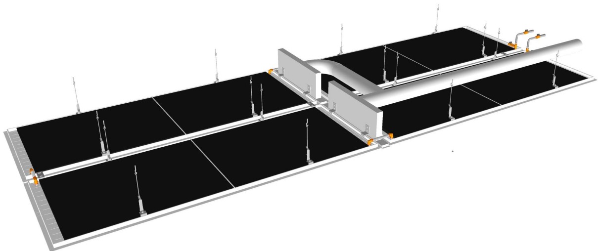
Fig. 2 – Ansicht der Rückseite der Deckensegel, Montageart mit Schnellabhängern, mit Akustik und optionaler integrierter Lüftung
