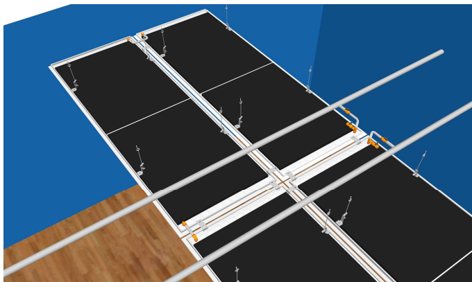
Fig. 8 - Standard Klimadecken mit Akustikdämmplatten
