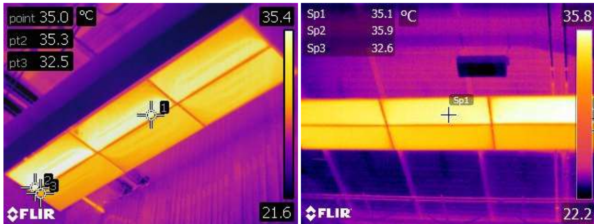
Fig. 5 - Die Infrarotbilder zeigen eindeutig wenn die KIGO Platten nicht vollständig durchströmt werden
