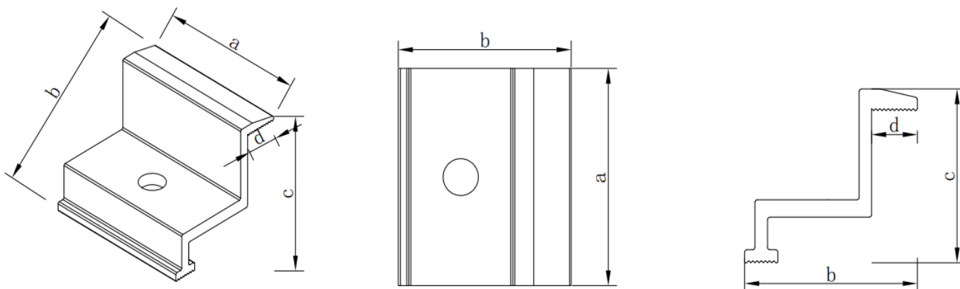
Fig. 5 Clamp
