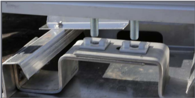
Einsetzen durch die Nutensteine in den Befestigungspunkt
