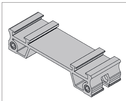
Pince à plier de notre propre production
